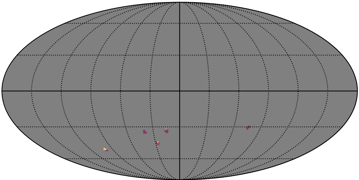
baseline_v3.4_10yrs : GalplaneFootprintMetric_clementini_stellarpops_map_Tau_5_0
