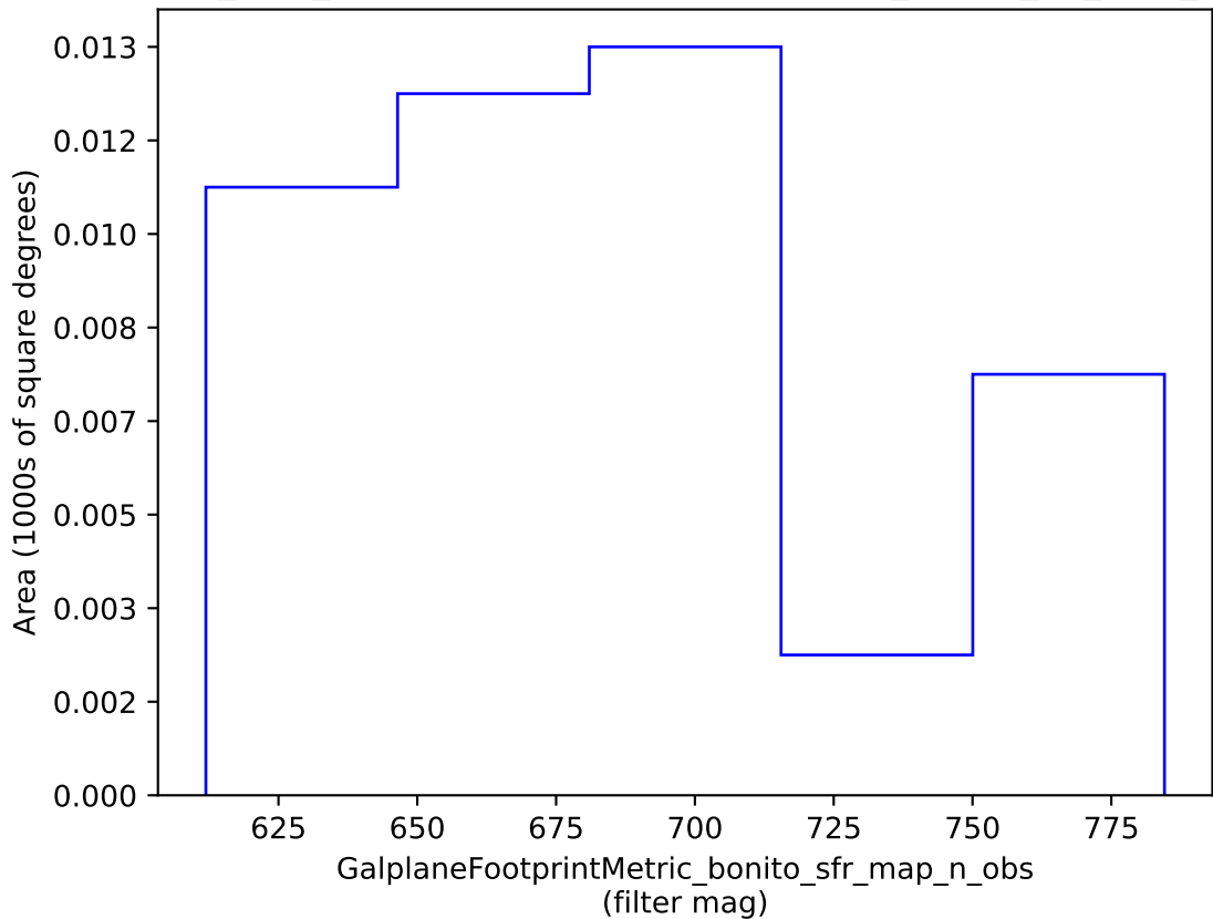
baseline_v3.4_10yrs : GalplaneFootprintMetric_bonito_sfr_map_n_obs
