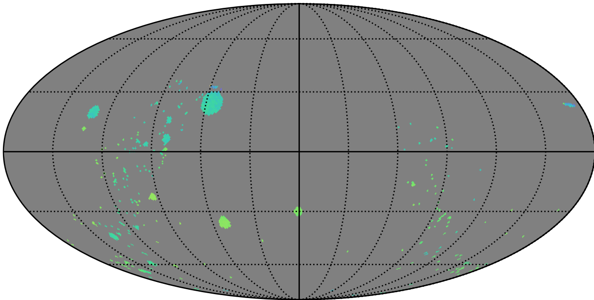
baseline_v3.4_10yrs : GalPlaneVisitIntervalsTimescales_open_clusters_map_Tau_2_0
