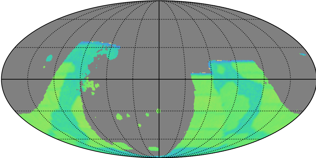
baseline_v3.4_10yrs : GalPlaneVisitIntervalsTimescales_combined_map_Tau_2_0
