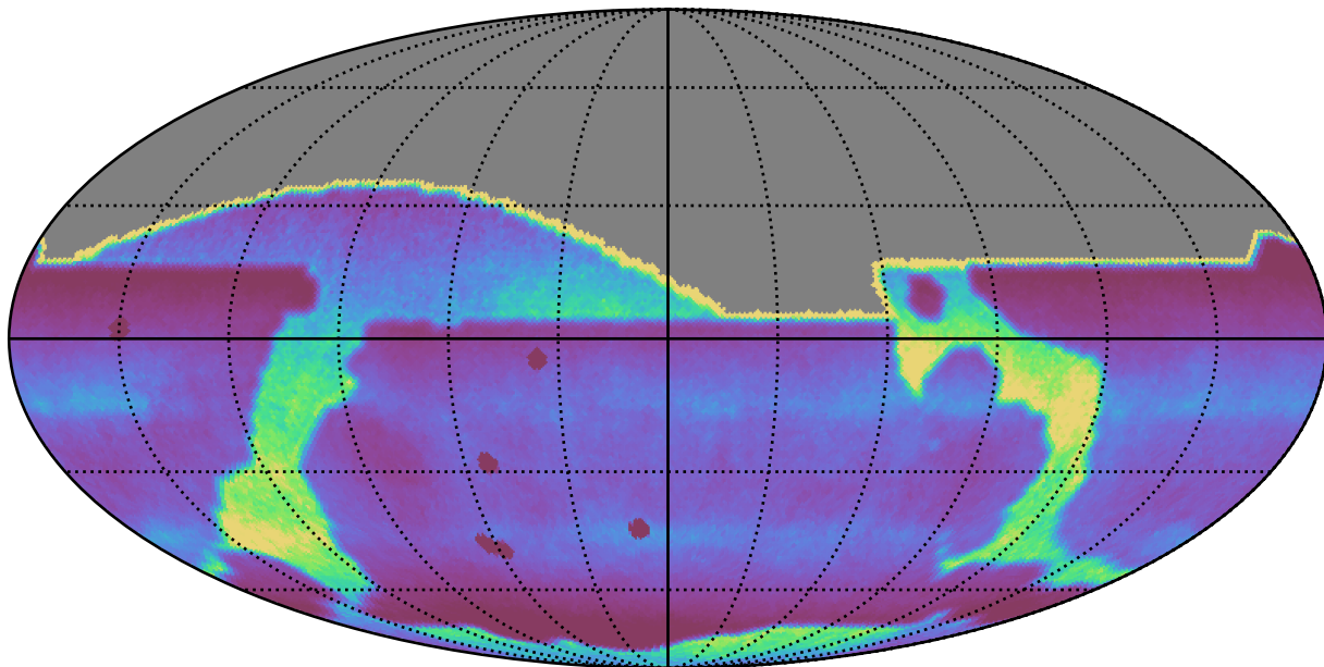
baseline_v3.4_10yrs : DCRprecision
