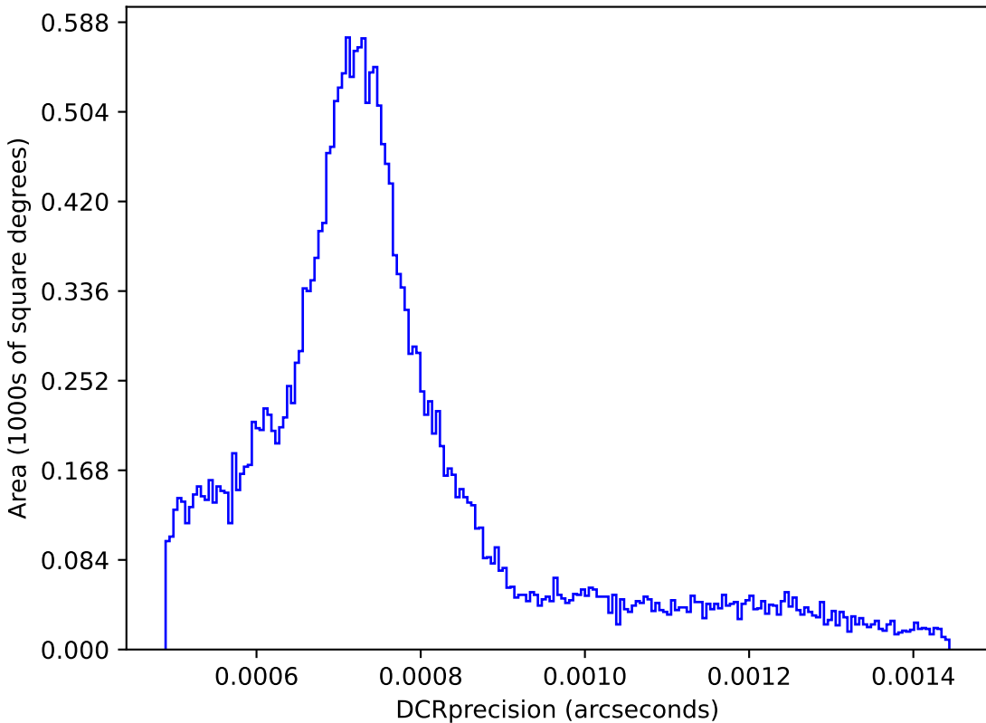
baseline_v3.4_10yrs : DCRprecision
