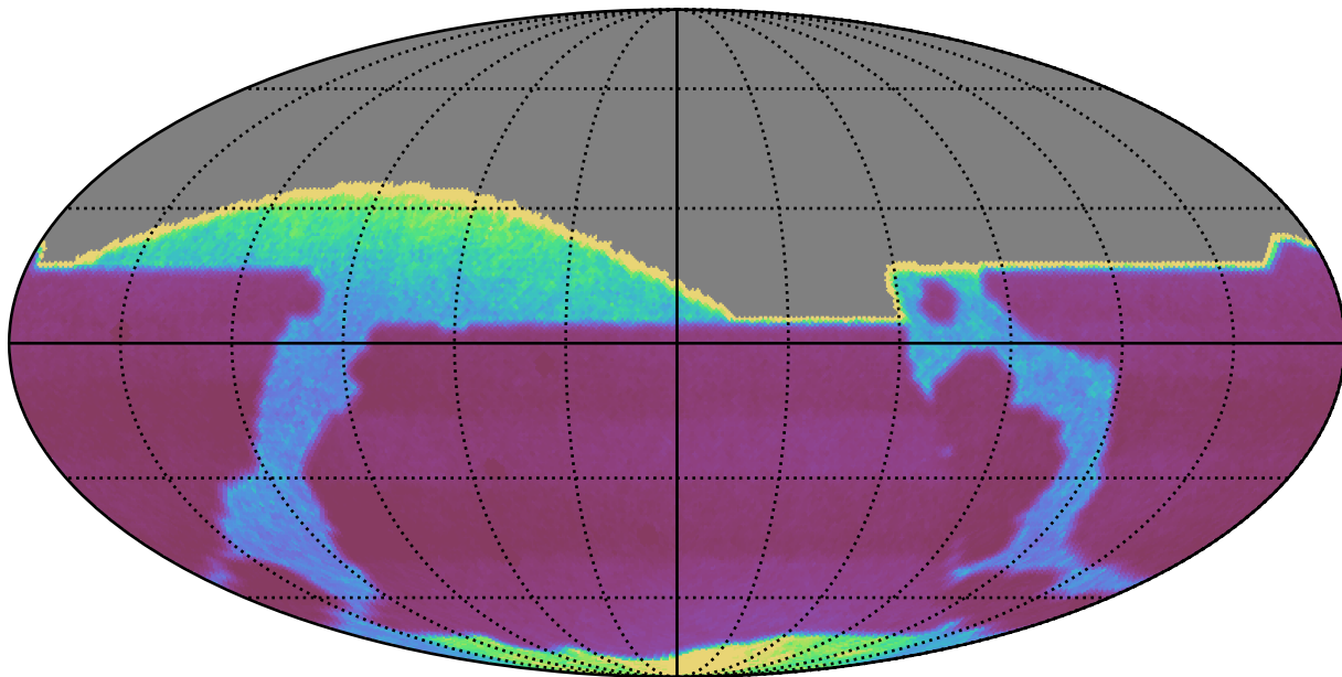
baseline_v3.4_10yrs : properMotion
