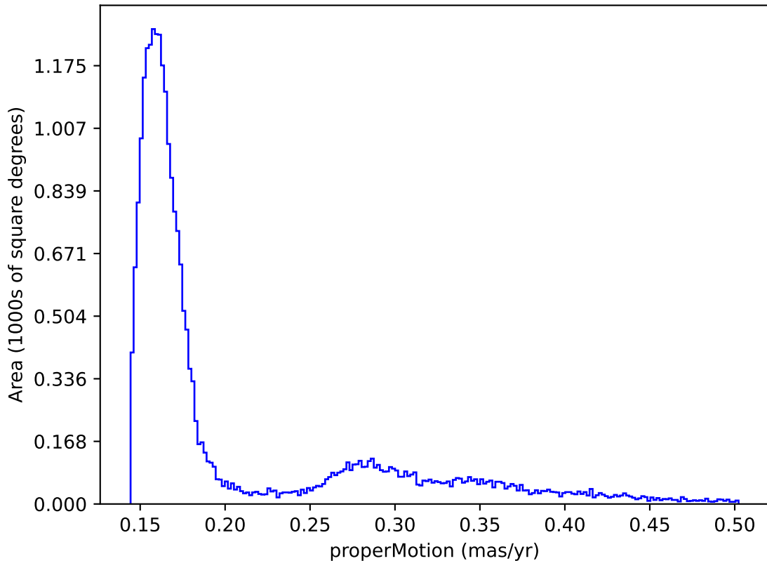
baseline_v3.4_10yrs : properMotion
