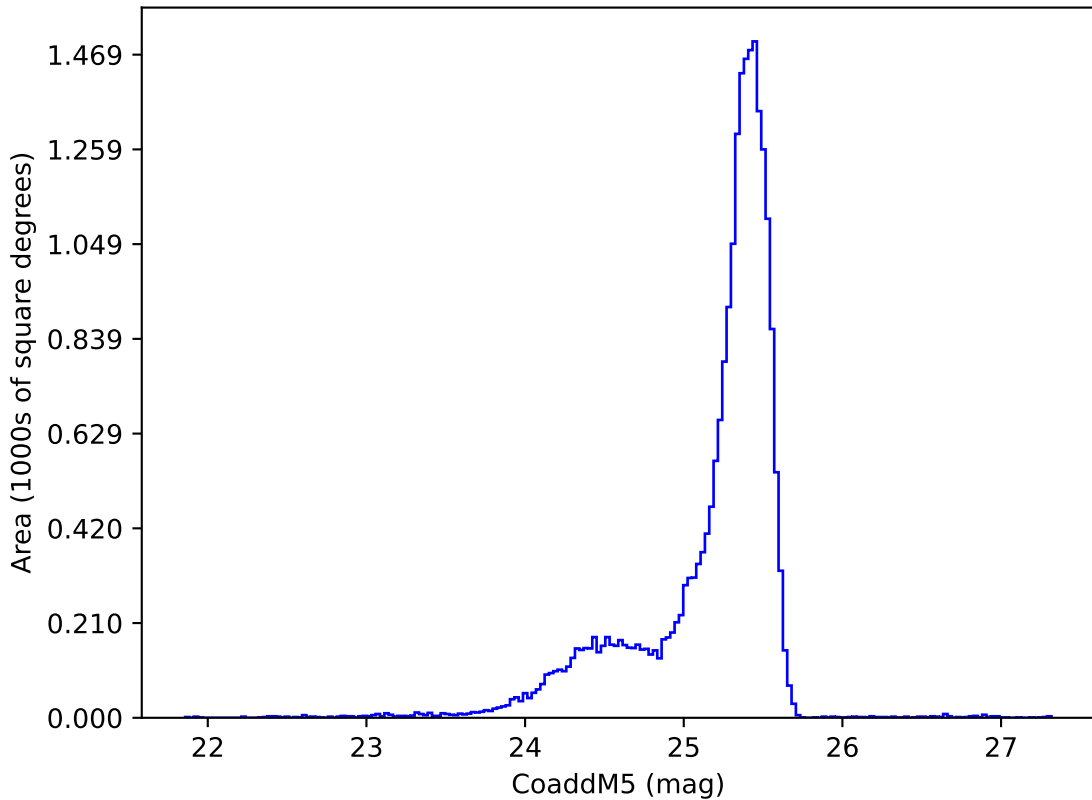
baseline_v3.4_10yrs u: CoaddM5
