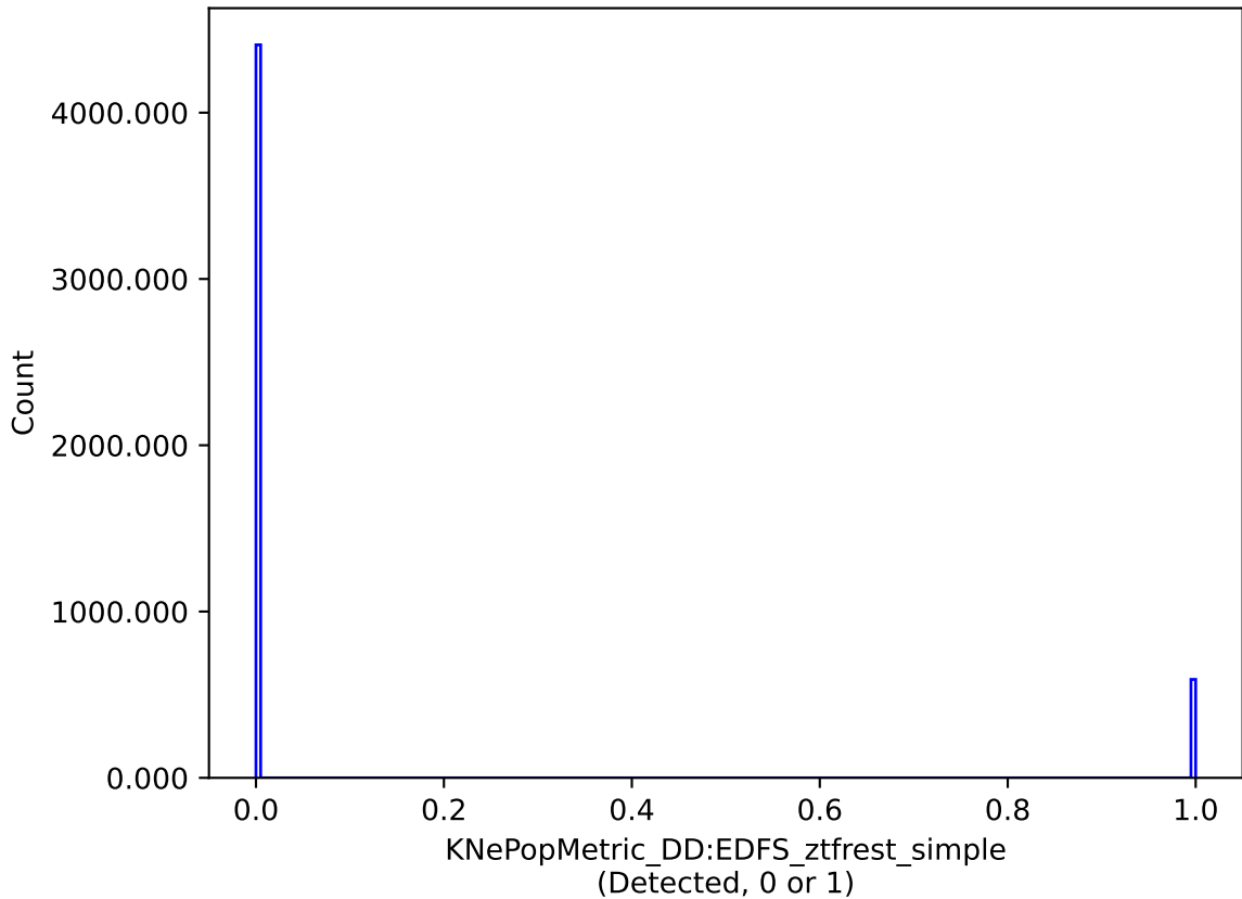
baseline_v3.4_10yrs DD:EDFS: KNePopMetric_DD:EDFS_ztfrest_simple
