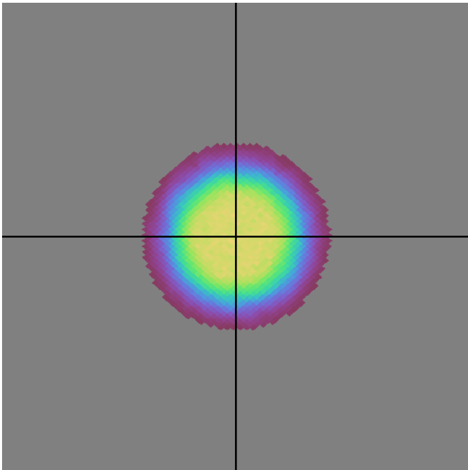
baseline_v3.4_10yrs r band: DD:XMM_LSS NVisits
