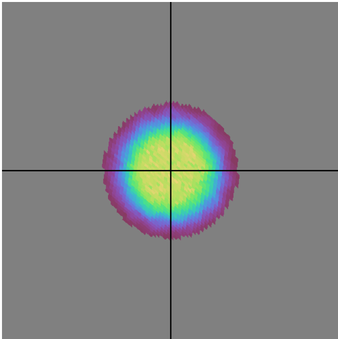
baseline_v3.4_10yrs u band: DD:ELAISS1 NVisits
