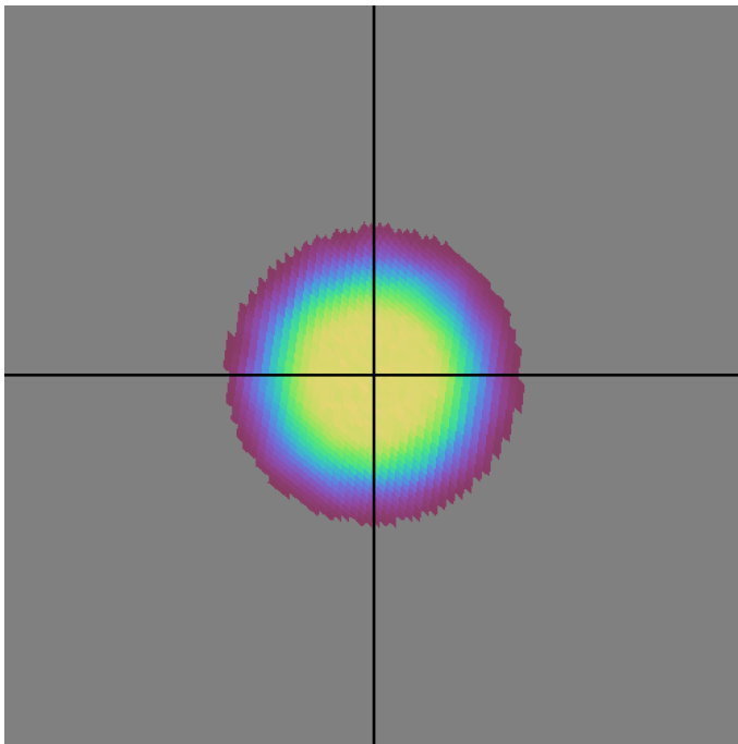
baseline_v3.4_10yrs all bands: DD:ELAISS1 NVisits
