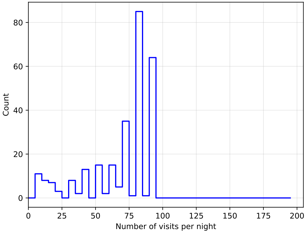
baseline_v3.4_10yrs all bands: DD:ELAISS1 NVisitsPerNight
