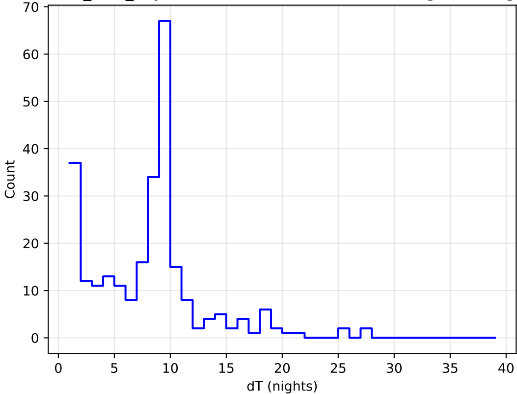
baseline_v3.4_10yrs all bands: DD:ELAISS1 Delta Nights Histogram
