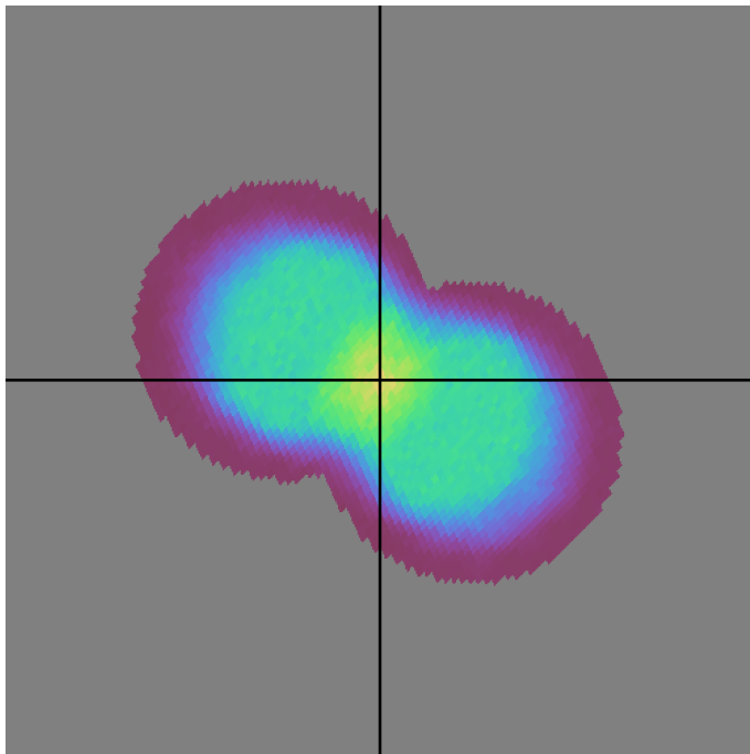
baseline_v3.4_10yrs u band: DD:EDFS NVisits
