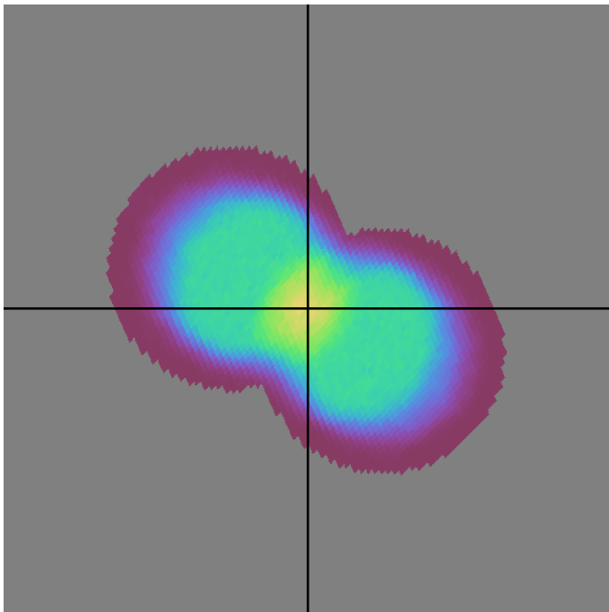
baseline_v3.4_10yrs r band: DD:EDFS NVisits
