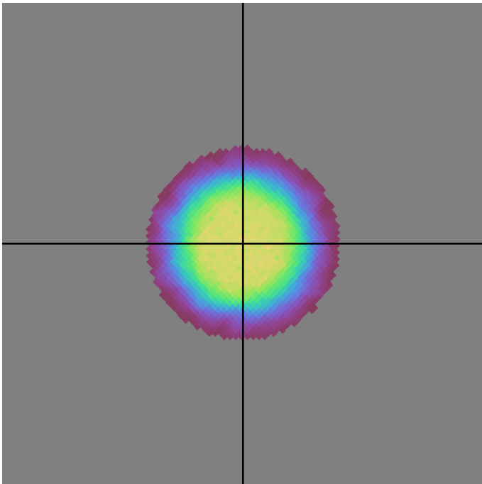
baseline_v3.4_10yrs z band: DD:ECDFS NVisits
