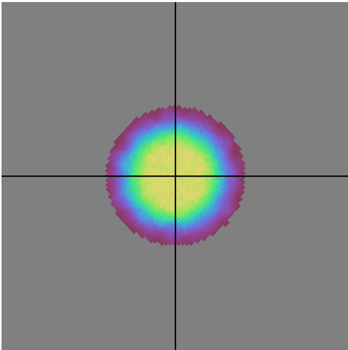
baseline_v3.4_10yrs g band: DD:ECDFS NVisits
