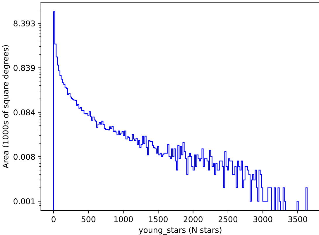
baseline_v3.3_10yrs : young_stars
