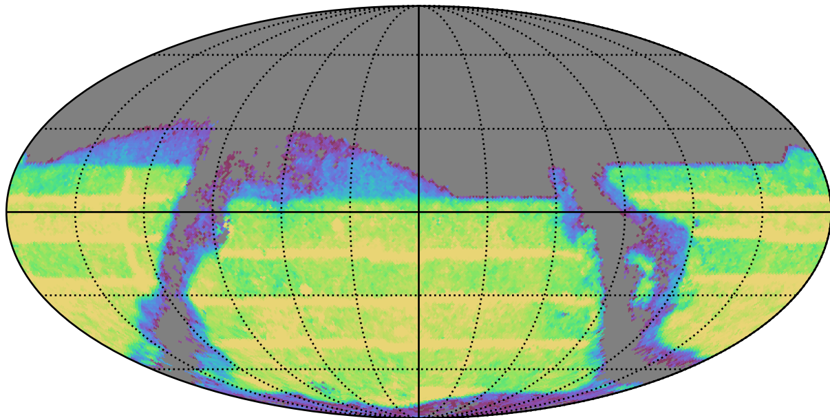
baseline_v3.3_10yrs : TDC_rate
