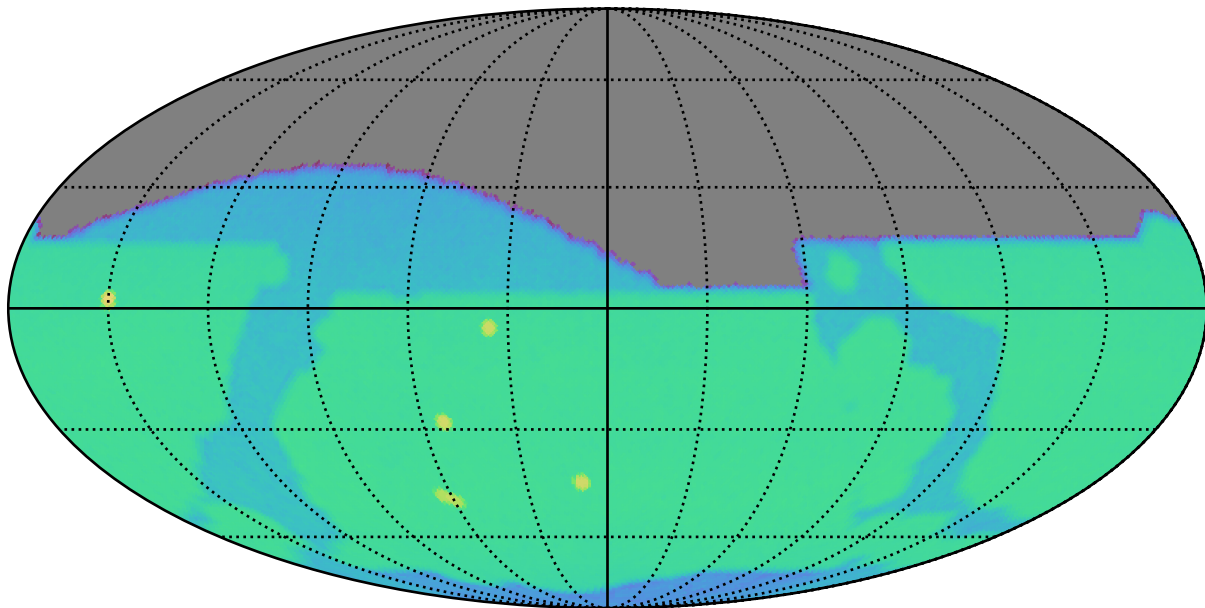
baseline_v3.3_10yrs i: SurfaceBrightLimit
