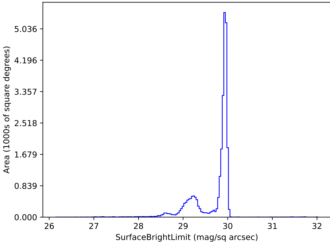
baseline_v3.3_10yrs i: SurfaceBrightLimit
