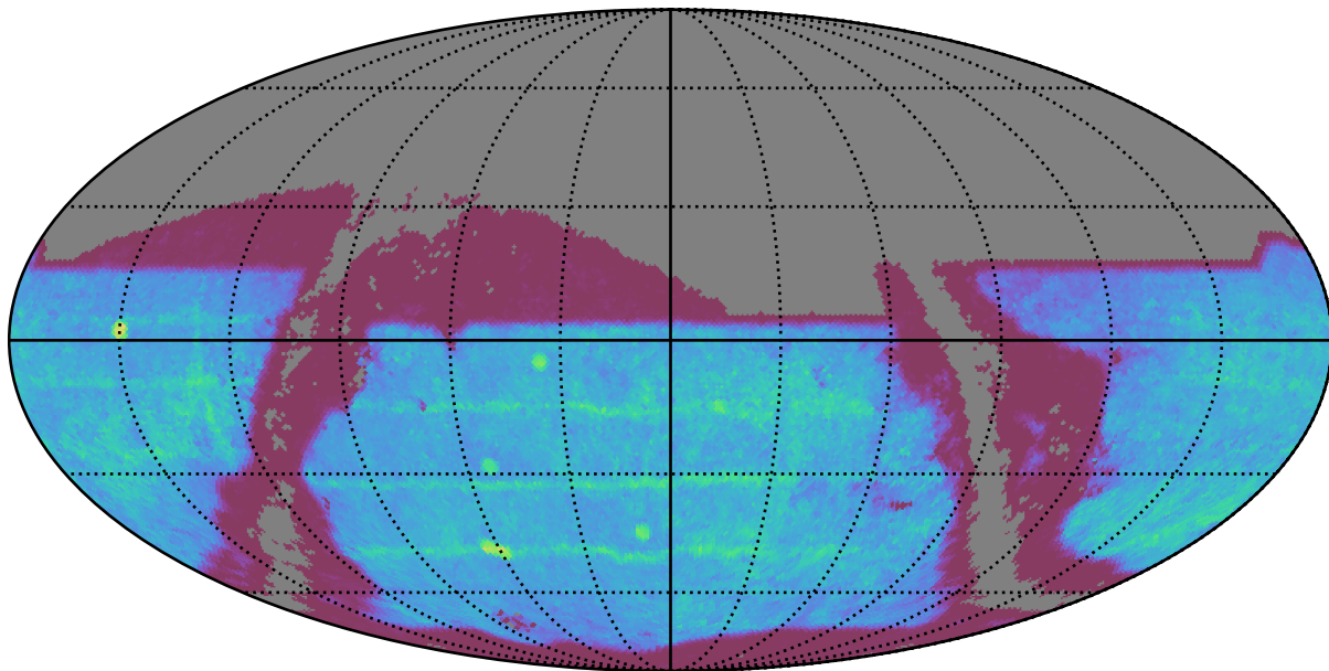
baseline_v3.3_10yrs : SNSLMetric
