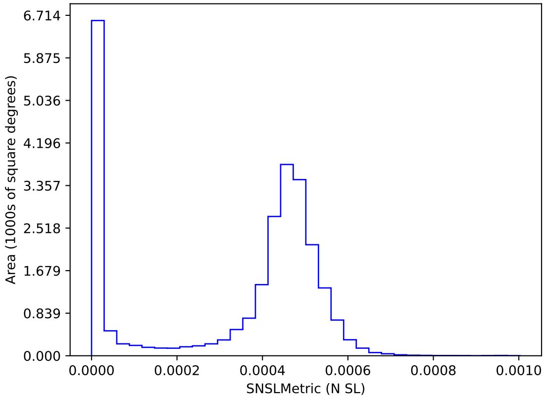
baseline_v3.3_10yrs : SNSLMetric
