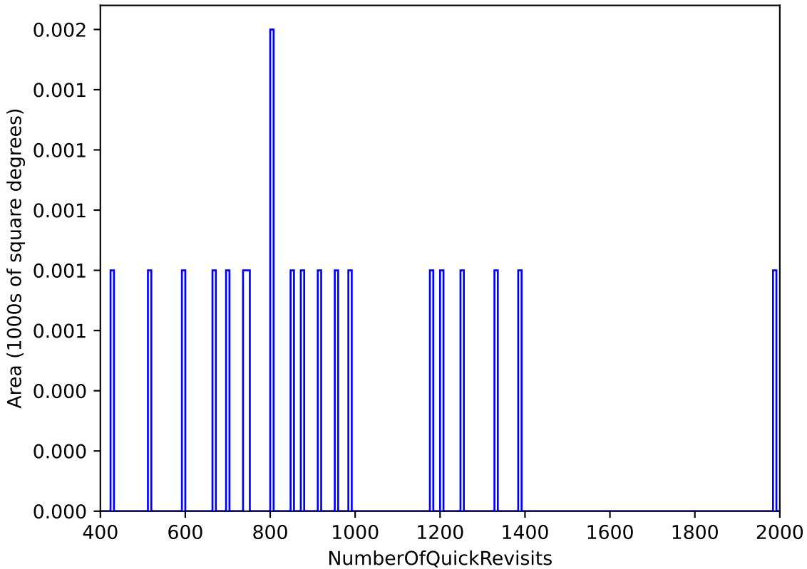
baseline_v3.3_10yrs : NumberOfQuickRevisits
