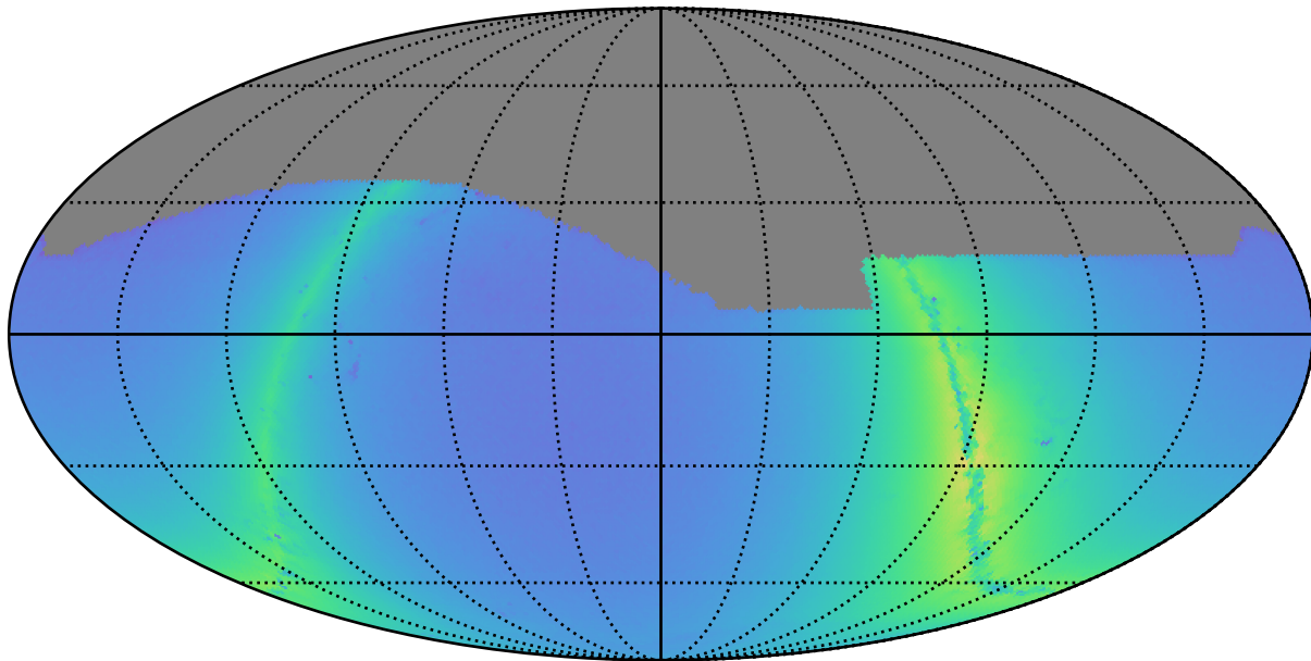
baseline_v3.3_10yrs i: Nstars_no_crowding
