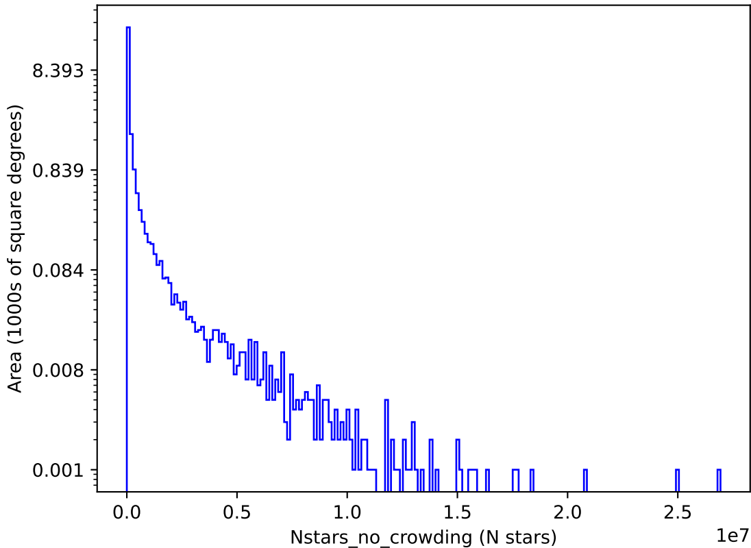
baseline_v3.3_10yrs i: Nstars_no_crowding
