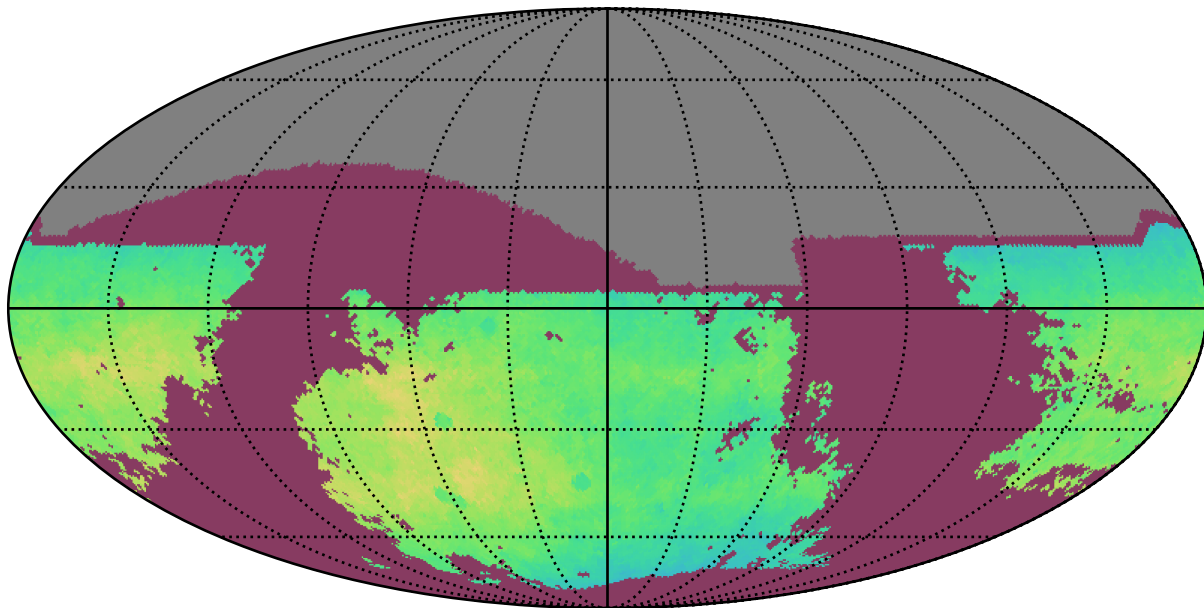
baseline_v3.3_10yrs i: NgalScale
