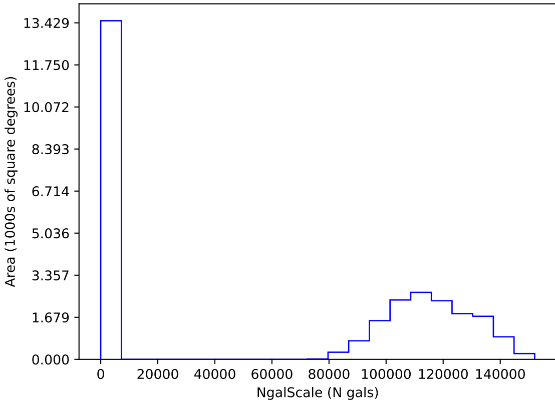
baseline_v3.3_10yrs i: NgalScale
