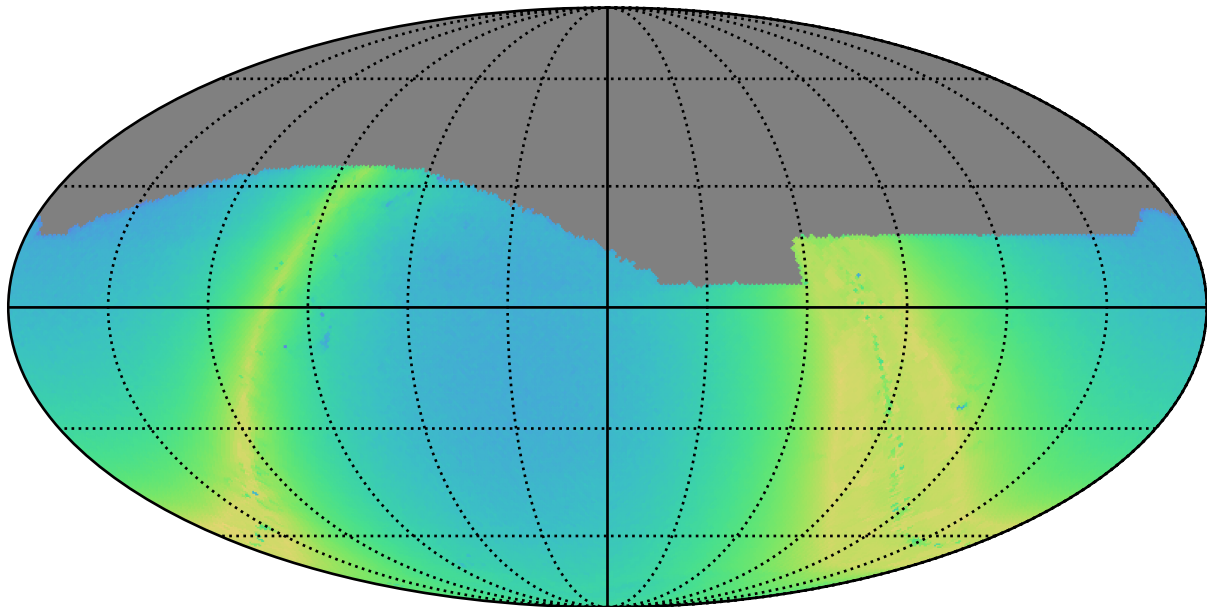
baseline_v3.3_10yrs i: N stars to Precision 0.20
