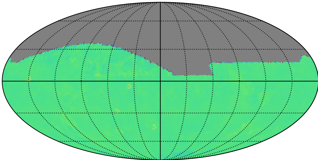
baseline_v3.3_10yrs z: Kuiper rotTelPos
