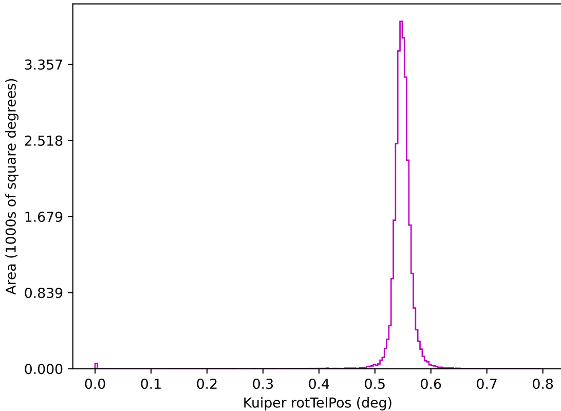
baseline_v3.3_10yrs z: Kuiper rotTelPos
