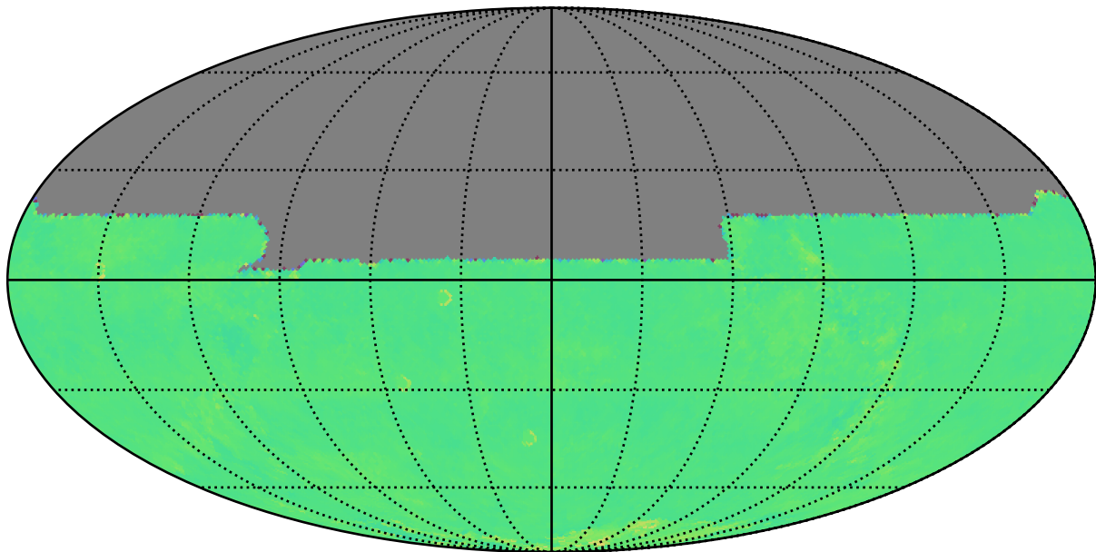
baseline_v3.3_10yrs y: Kuiper rotTelPos
