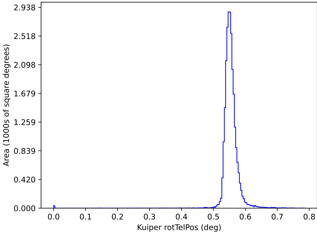
baseline_v3.3_10yrs y: Kuiper rotTelPos
