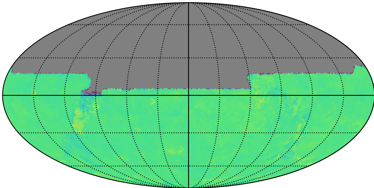
baseline_v3.3_10yrs u: Kuiper rotTelPos
