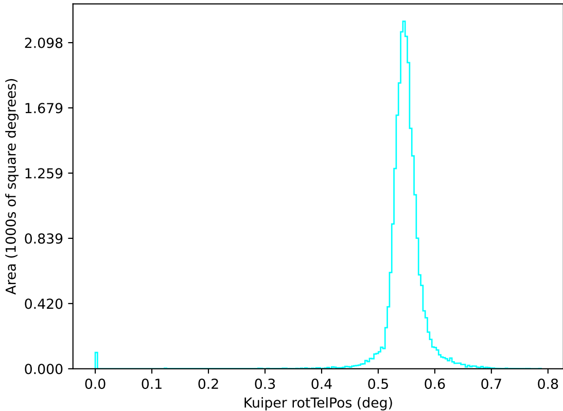
baseline_v3.3_10yrs u: Kuiper rotTelPos
