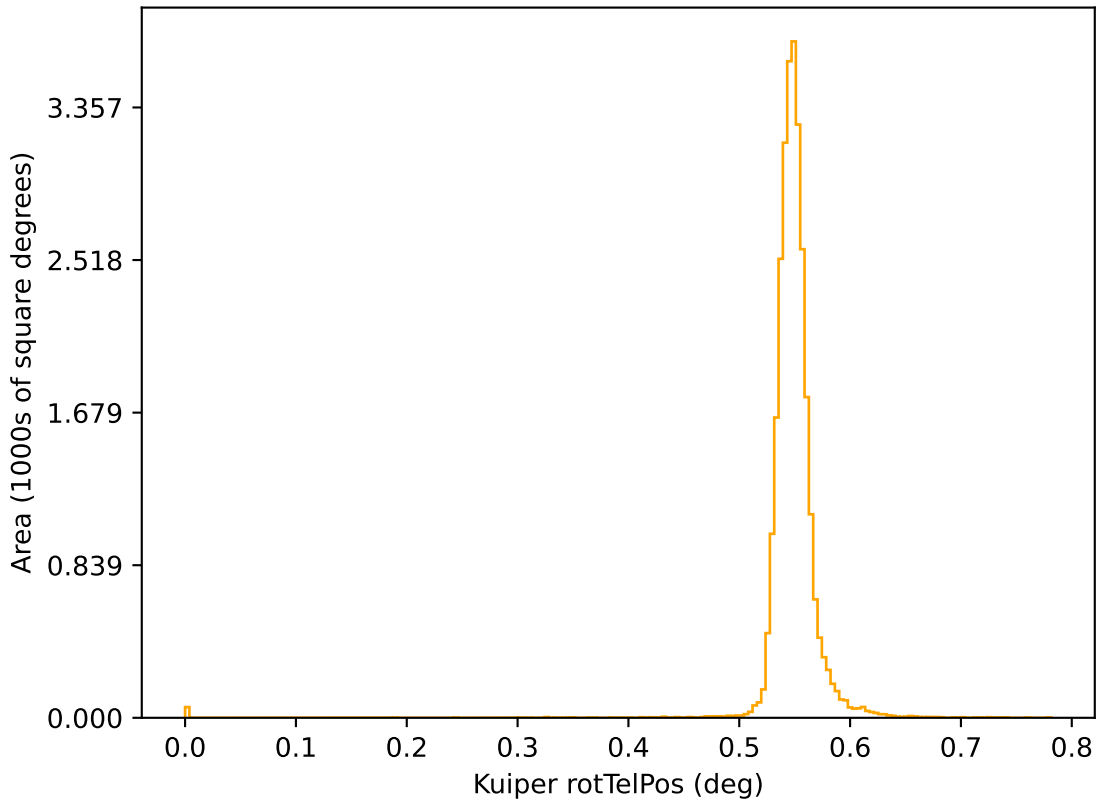
baseline_v3.3_10yrs r: Kuiper rotTelPos
