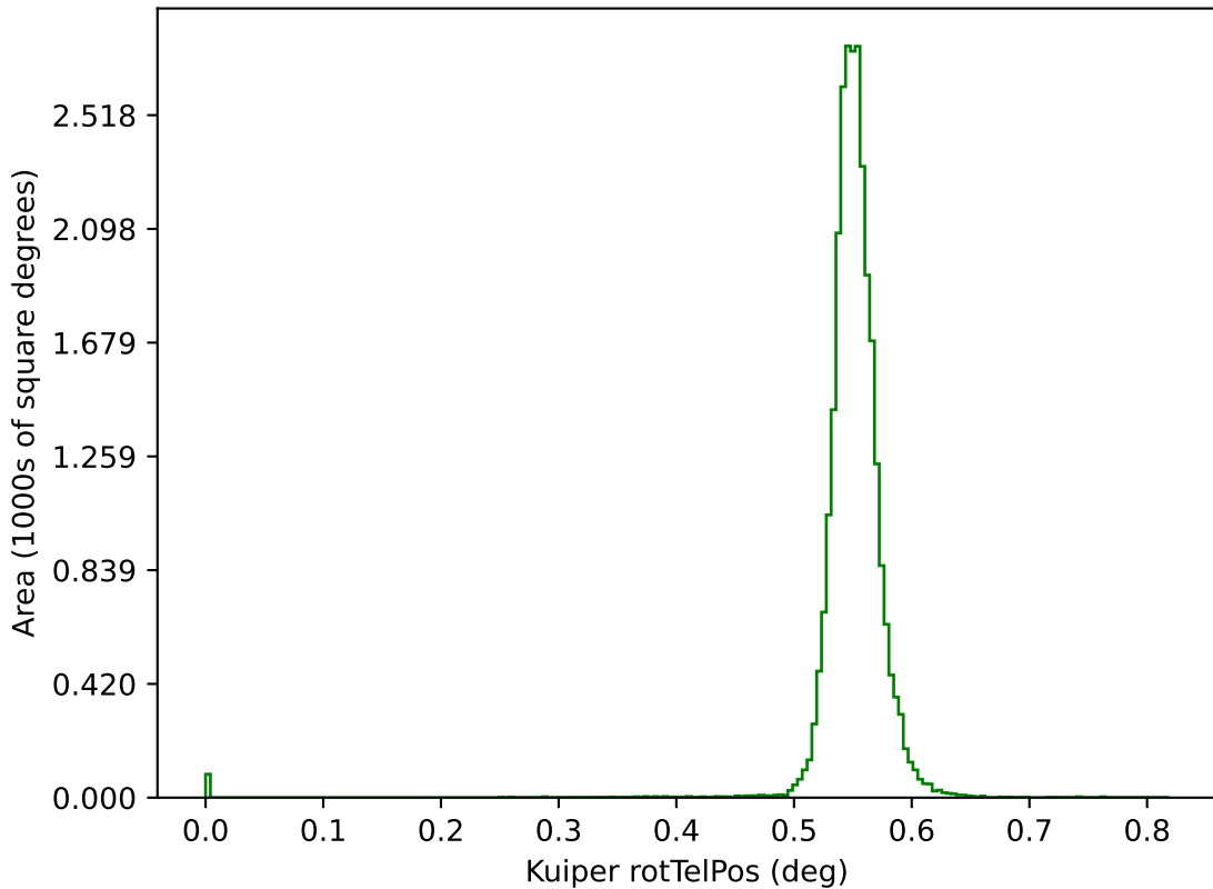
baseline_v3.3_10yrs g: Kuiper rotTelPos
