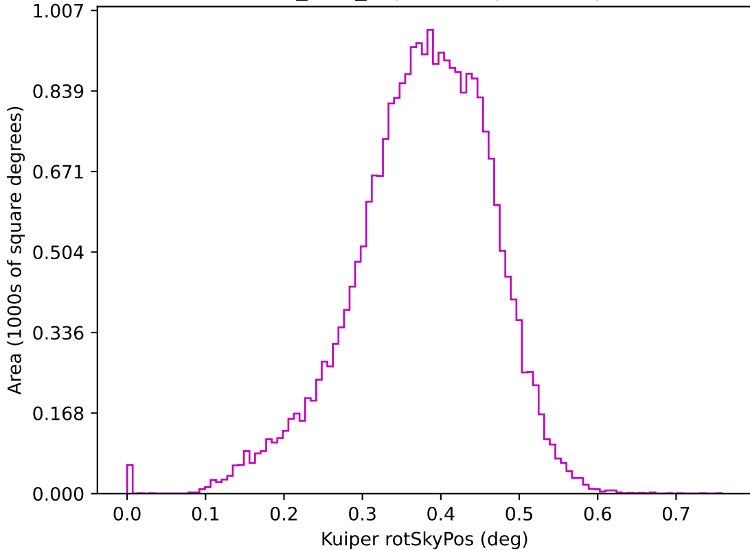
baseline_v3.3_10yrs z: Kuiper rotSkyPos
