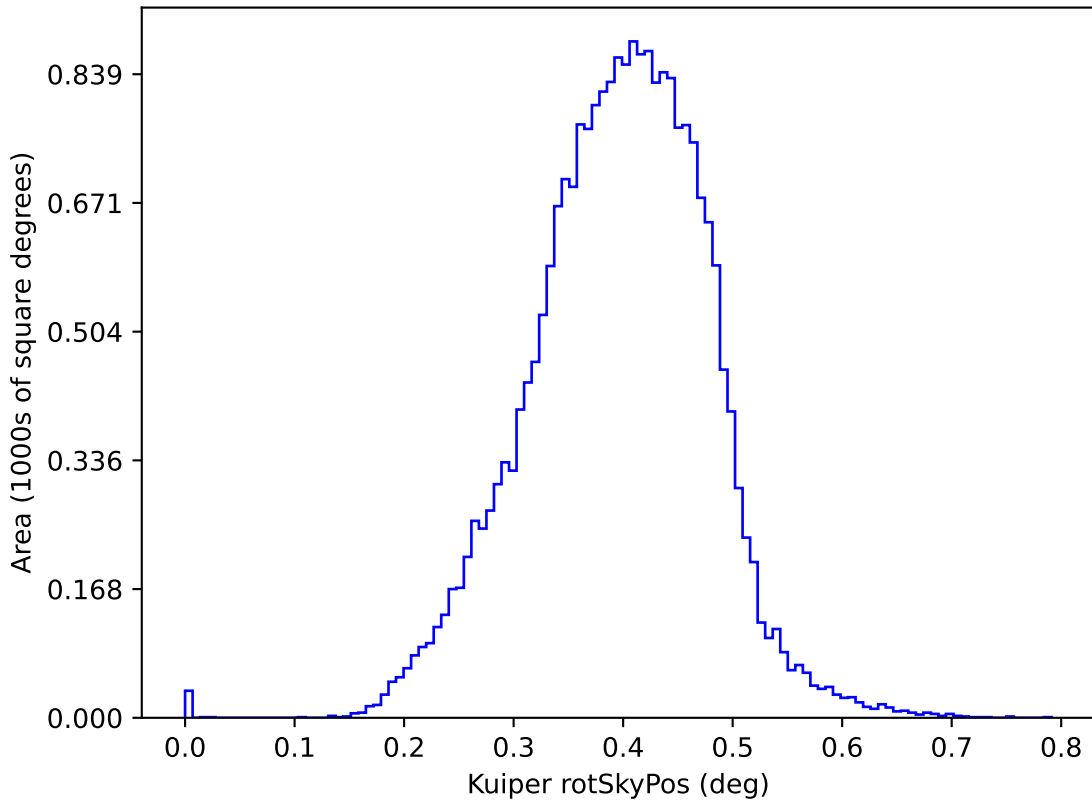
baseline_v3.3_10yrs y: Kuiper rotSkyPos
