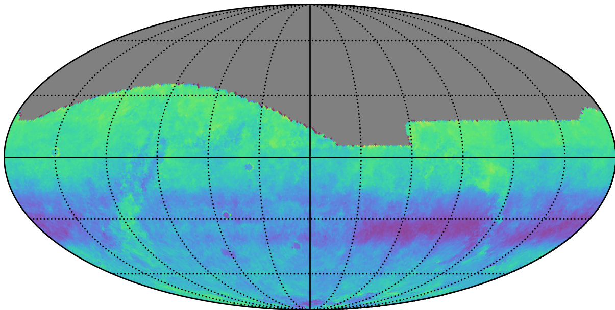
baseline_v3.3_10yrs r: Kuiper rotSkyPos
