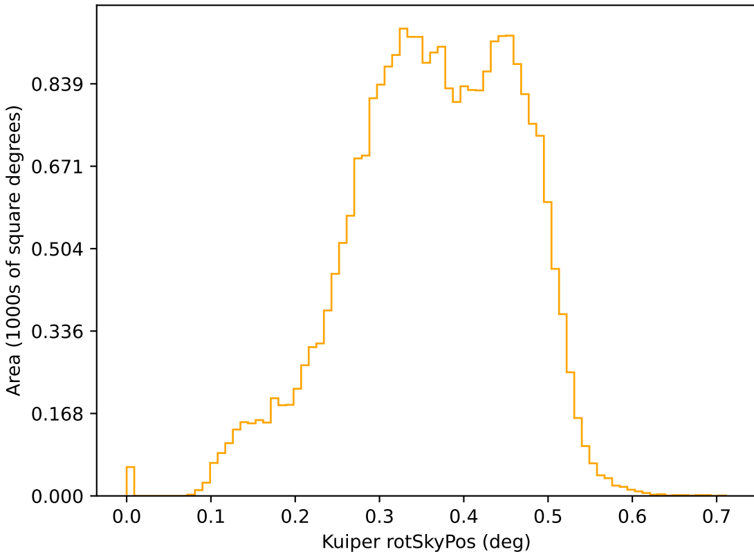
baseline_v3.3_10yrs r: Kuiper rotSkyPos
