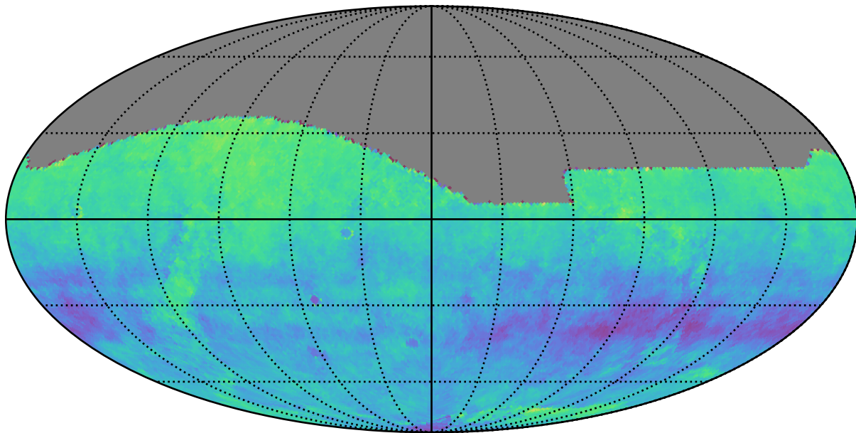
baseline_v3.3_10yrs i: Kuiper rotSkyPos
