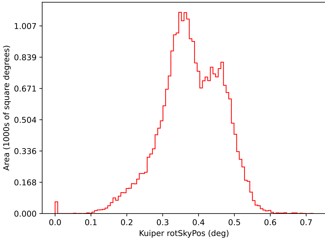
baseline_v3.3_10yrs i: Kuiper rotSkyPos
