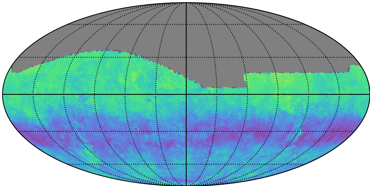
baseline_v3.3_10yrs g: Kuiper rotSkyPos
