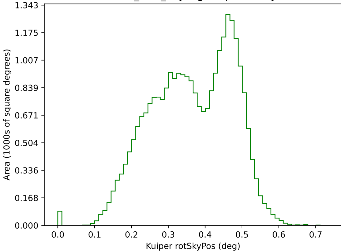
baseline_v3.3_10yrs g: Kuiper rotSkyPos
