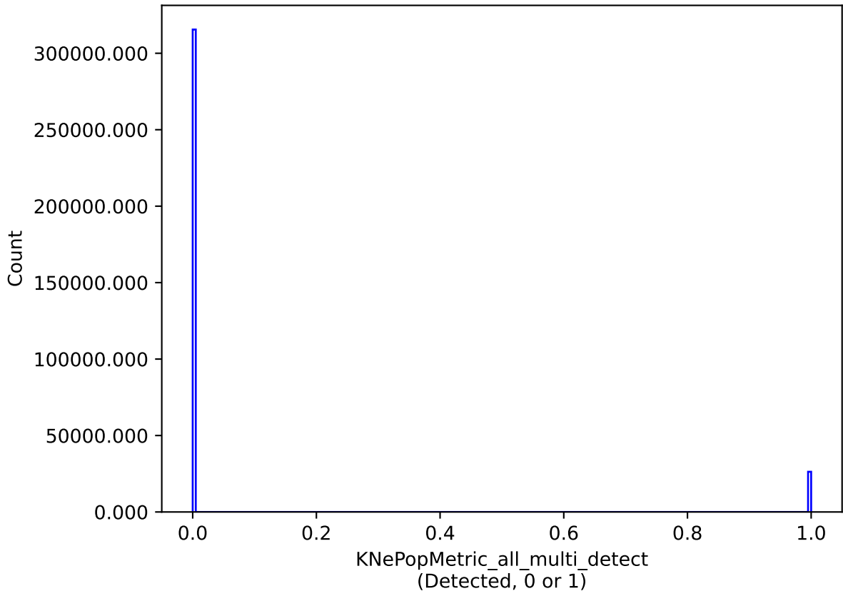
baseline_v3.3_10yrs all models: KNePopMetric_all_multi_detect
