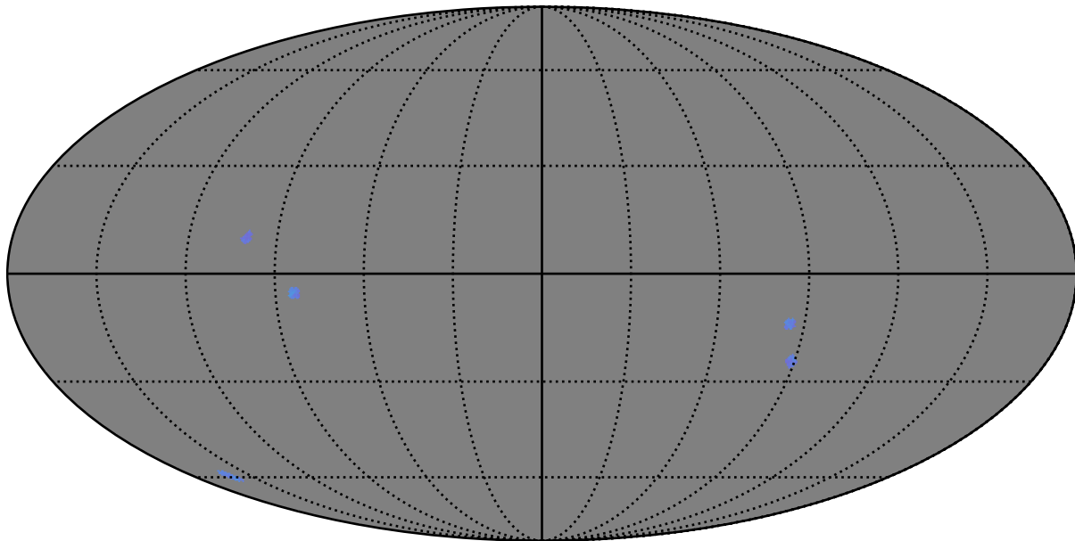
baseline_v3.3_10yrs : GalplaneTimePerFilter_bonito_sfr_map_g
