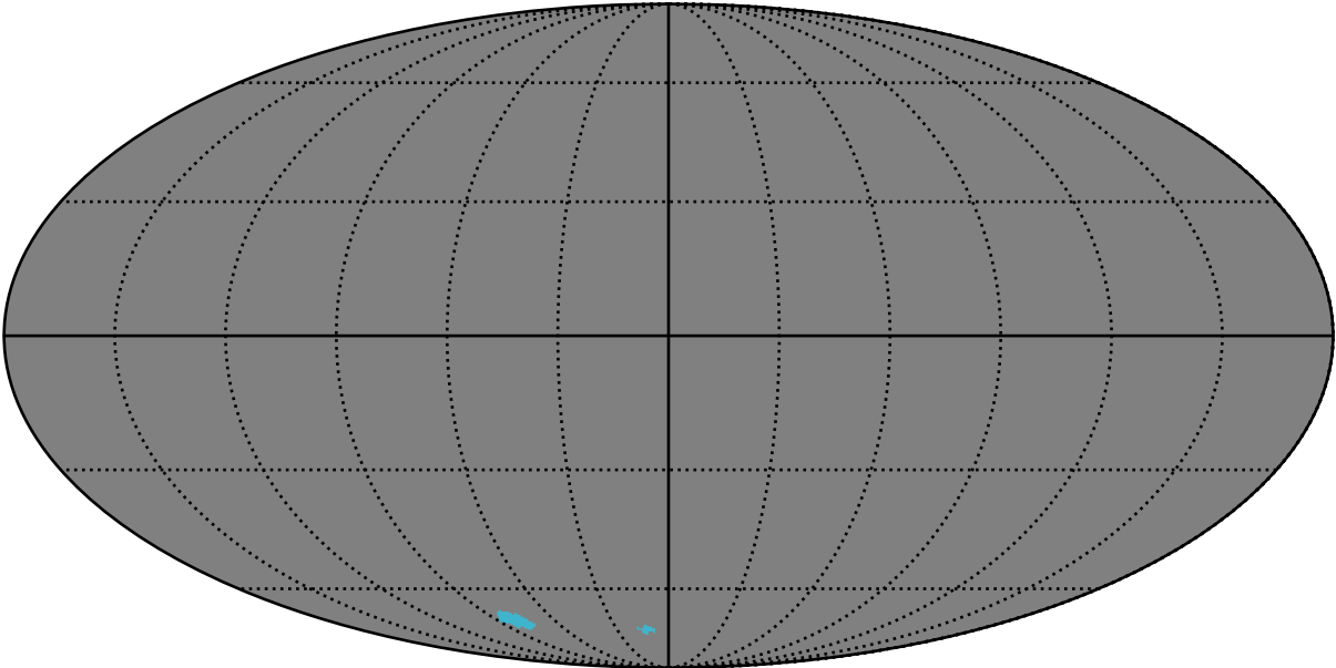
baseline_v3.3_10yrs : GalplaneFootprintMetric_magellanic_clouds_map_Tau_5_0
